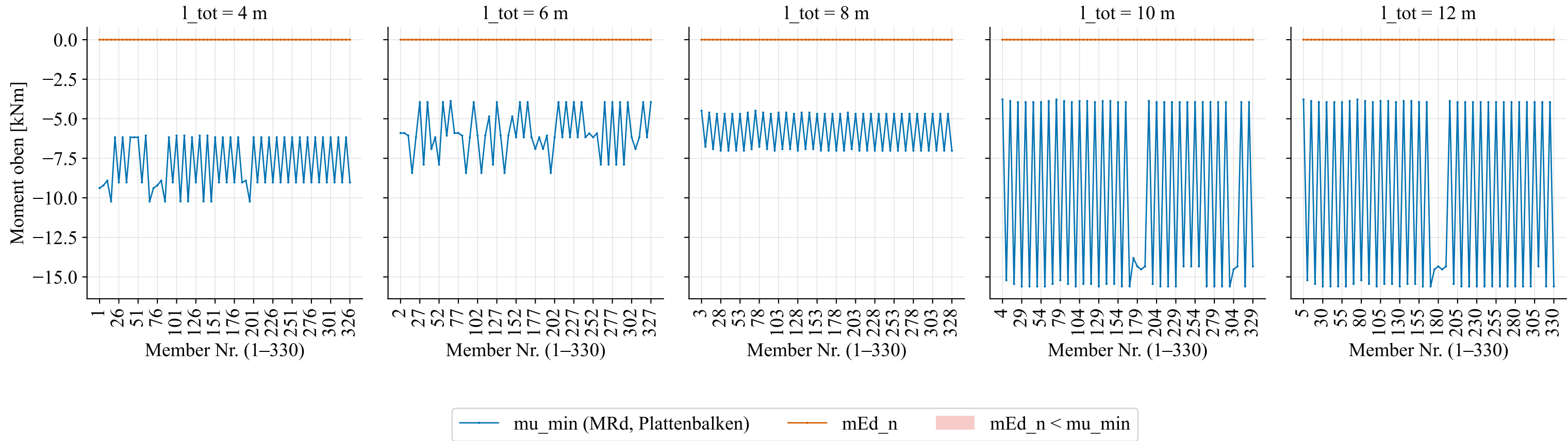
Biege widerstand \mu_{\min} (MRd, Plattenbalken) vs. Bemessungsmoment mEd_n je Member, kategorisiert nach Spannweite (Members_rc_rib_simple_)
